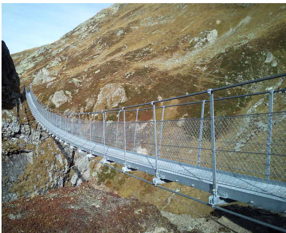
Die 60 m lange Hängebrücke Punt la Greina ist mit Blechprofilrost vom Typ Serrated belegt.
